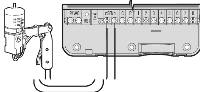
Mini-Cliik® Rain Sensor
